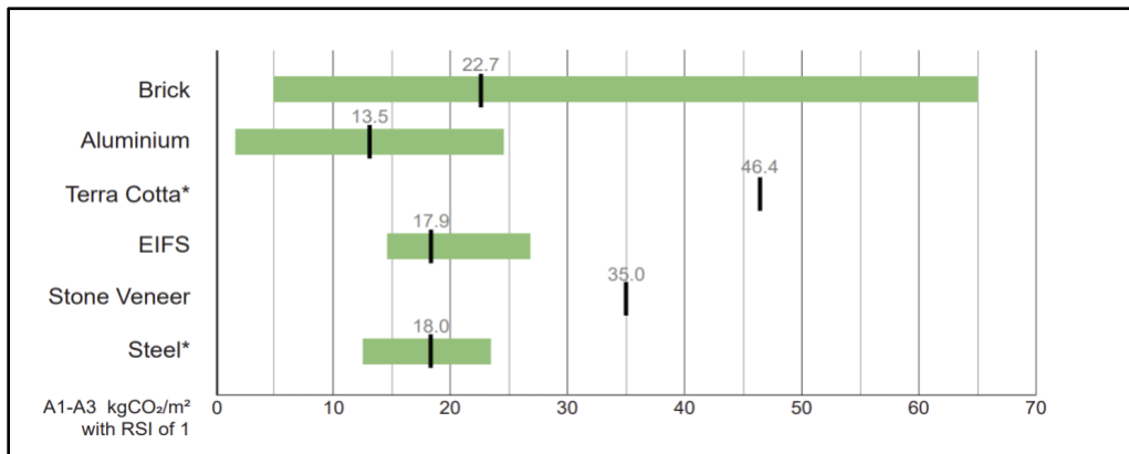
Figure 6 : Comparaison des émissions intrinsèques des produits de revêtement pour les étapes A1-A3 29
