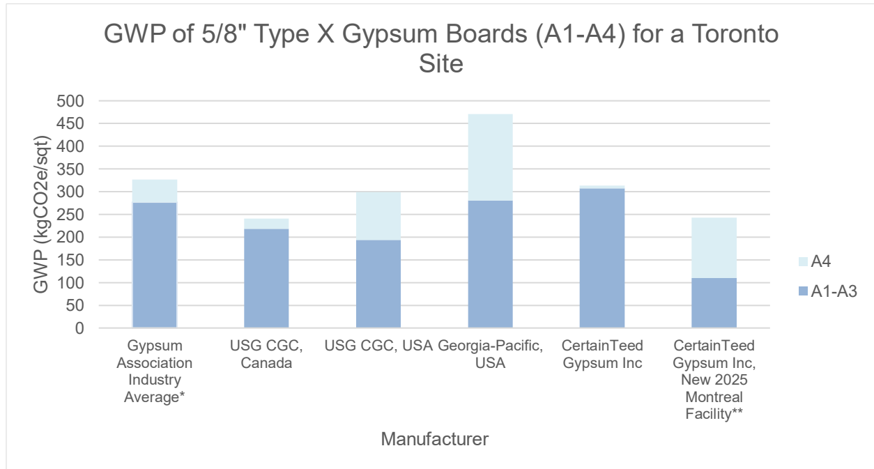
Figure 11 : Comparaison du potentiel de réchauffement planétaire (PRP) des panneaux de gypse de Type X de 5/8 po acheminés sur un chantier à Toronto (A1-A4)
