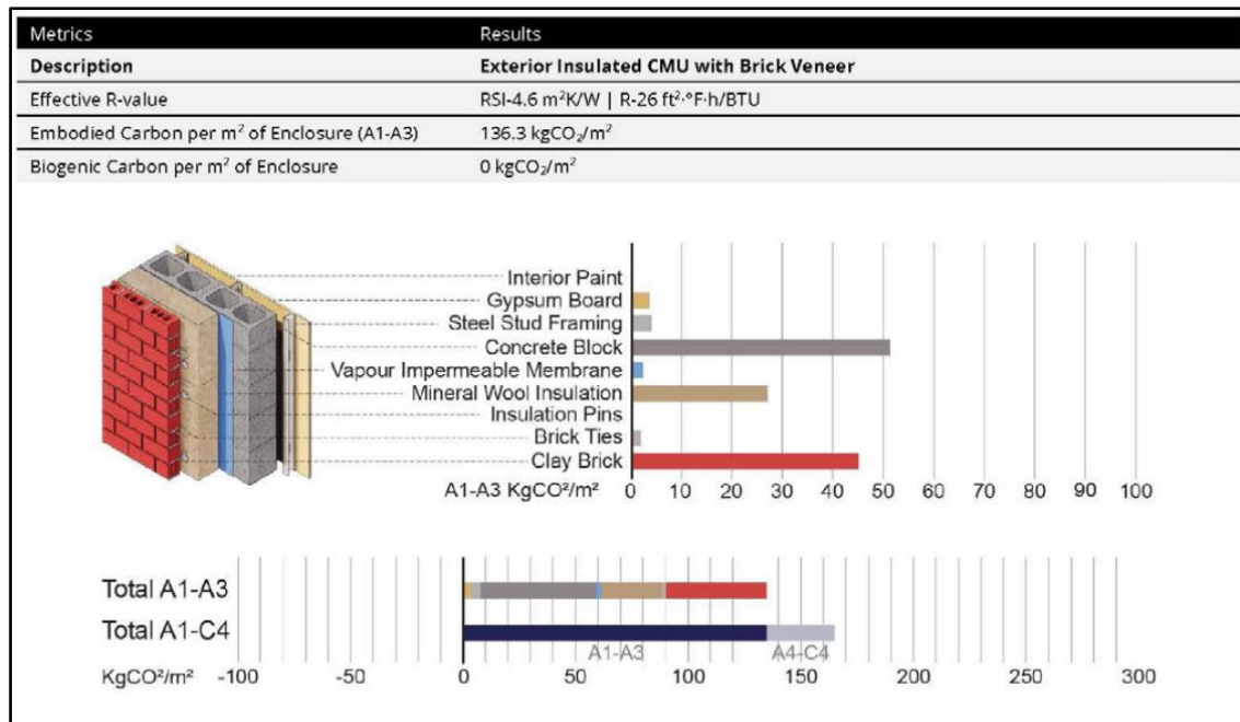
Figure 5 : Répartition des matériaux et du PRP d'un assemblage de mur typique -CMU isolé par l'extérieur avec parement de brique 28
