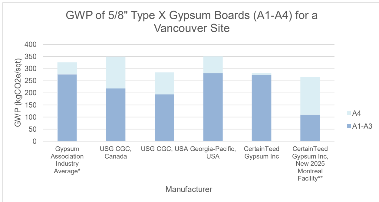
Figure 12 : Comparaison du potentiel de réchauffement planétaire (PRP) des panneaux de gypse de Type X de 5/8 po acheminés sur un chantier à Vancouver (A1-A4)
