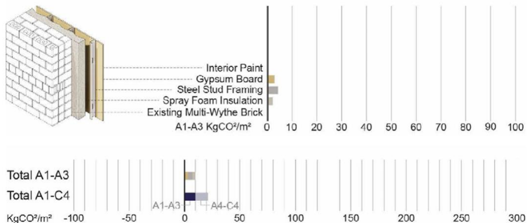
Figure 8 : Répartition des matériaux et du PRP d'un mur rénové - maçonnerie existante avec isolation intérieure en mousse pulvérisée 28
