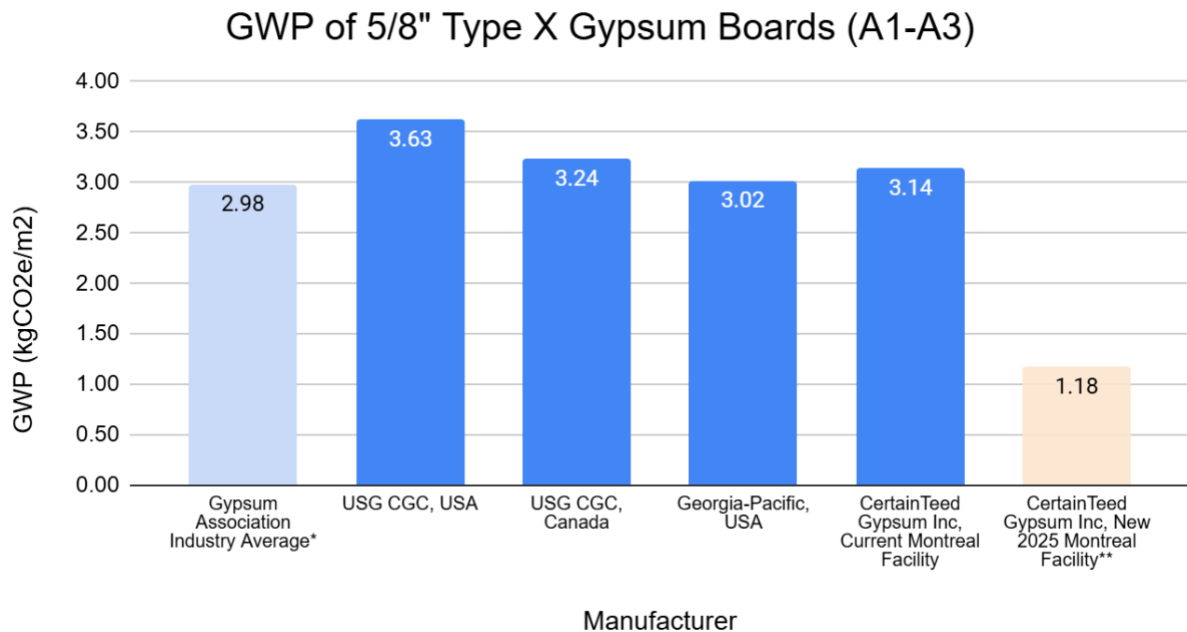
Figure 2 : Comparaison du potentiel de réchauffement planétaire (PRP) des panneaux de gypse de type X de 5/8 po de certaines entreprises nord-américaines
