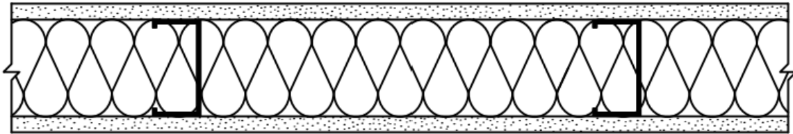
Figure 9 : Assemblage de mur intérieur résistant au feu pendant 1 heure avec montants en acier et isolation en fibre de verre (ULC U411) 32
