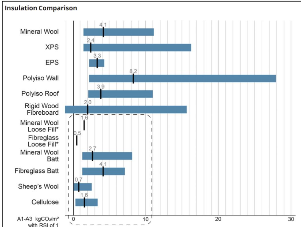
Figure 7 : Comparaison des émissions intrinsèques des matériaux isolants pour les étapes A1-A3 30
