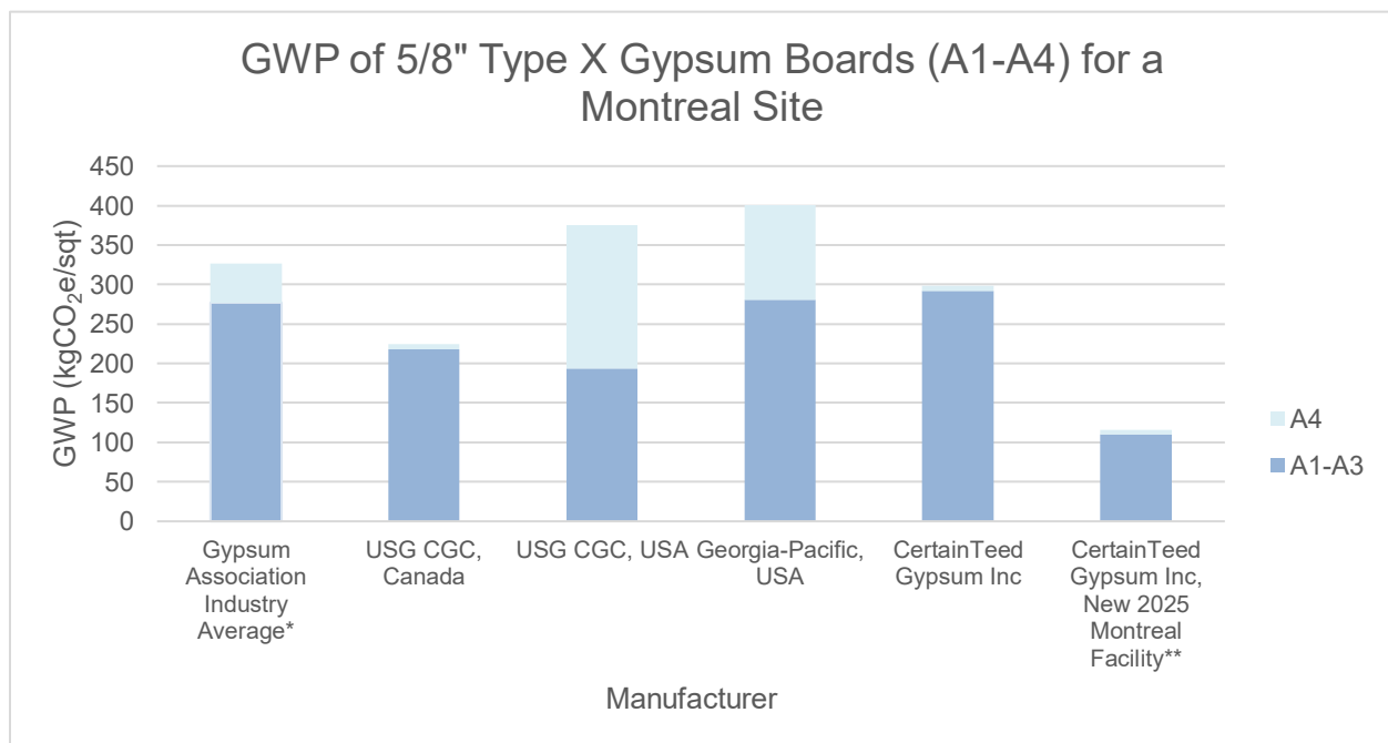
Figure 10 : Comparaison du potentiel de réchauffement planétaire (PRP) des panneaux de gypse de Type X de 5/8 po acheminés sur un chantier à Montréal (A1-A4)
