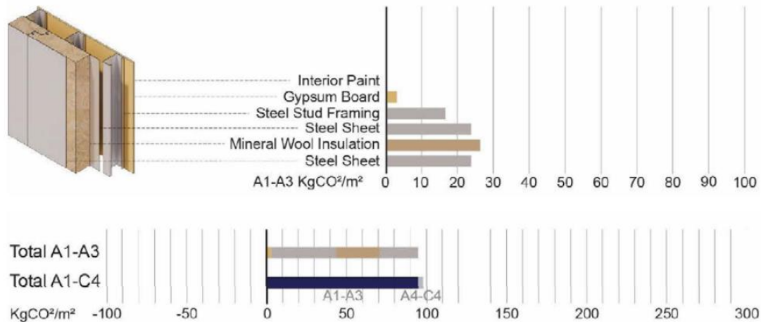
Figure 15 : assemblage mural typique : panneau métallique isolé avec isolation en laine minérale 28
