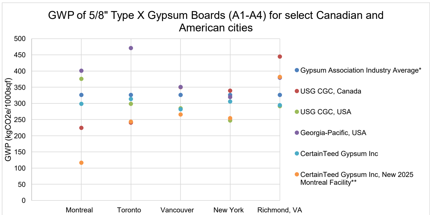
Figure 3 : Comparaison du potentiel de réchauffement planétaire (PRP) des panneaux de gypse de Type X de 5/8 po de certaines villes canadiennes et américaines (A1-A4)
