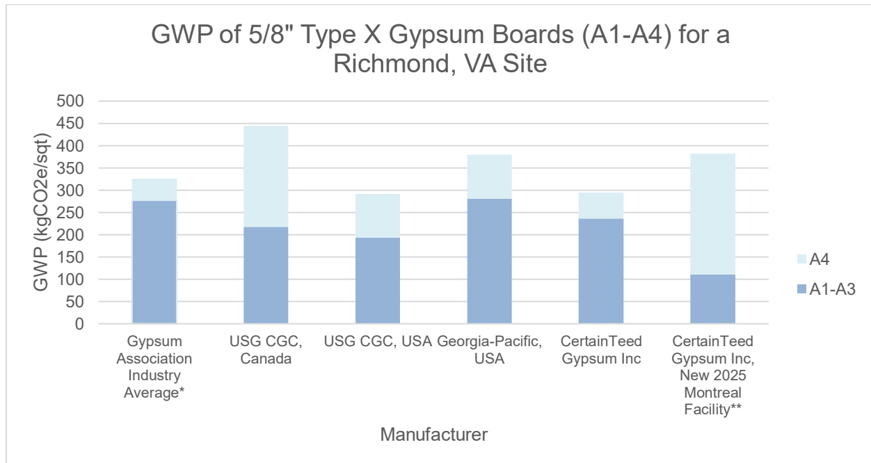
Figure 14 : Comparaison du potentiel de réchauffement planétaire (PRP) des panneaux de gypse de Type X de 5/8 po acheminés sur un chantier à Richmond, VA (A1-A4)
